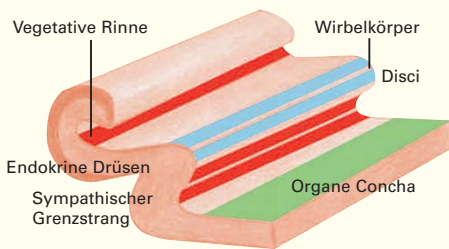
Transversaler Ohrquerschnitt
